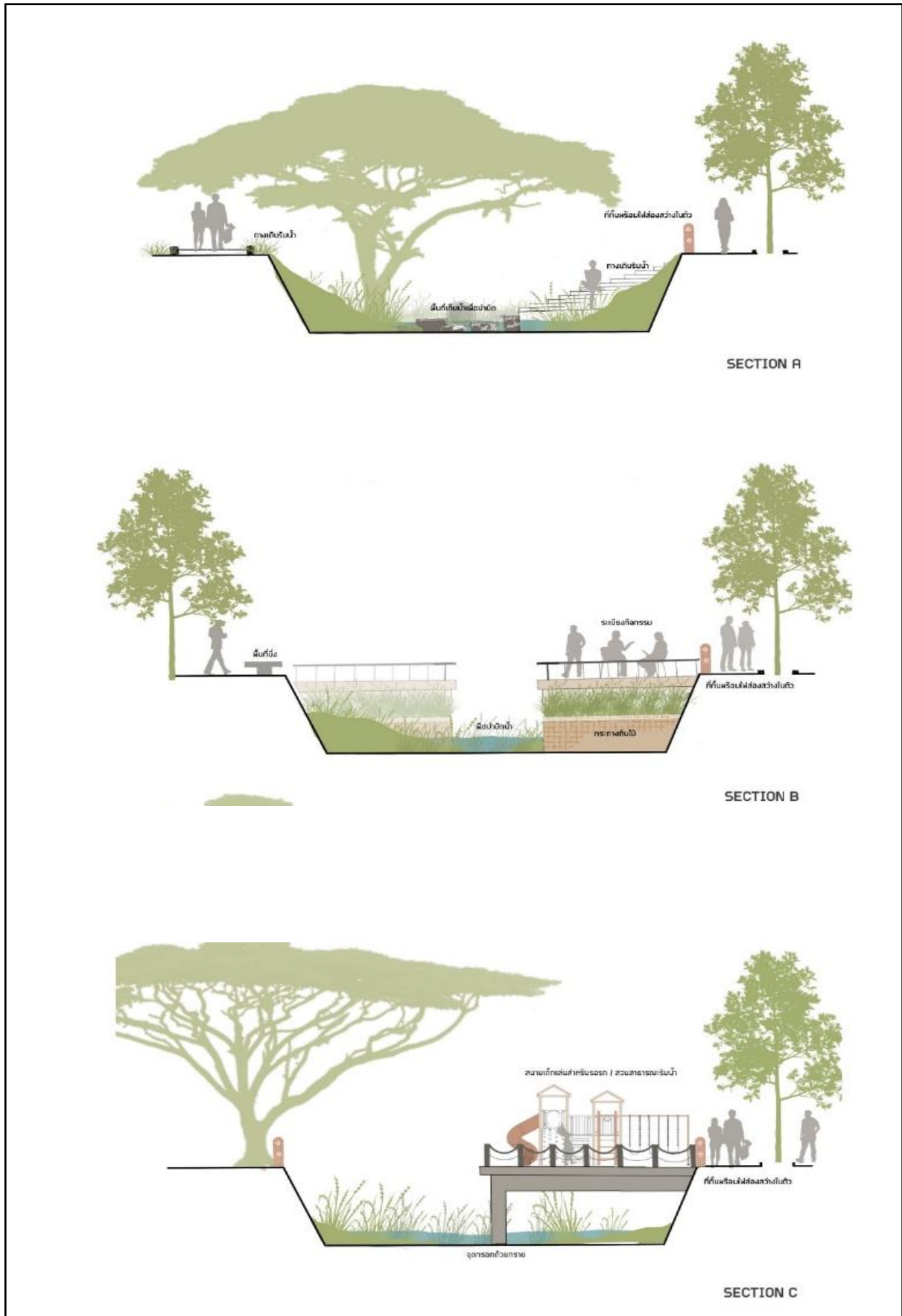
ภาพที่ ๑๓ รูปตัดแสดงรูปแบบพื้นที่สิ่งแวดล้อมและระบบนิเวศ
